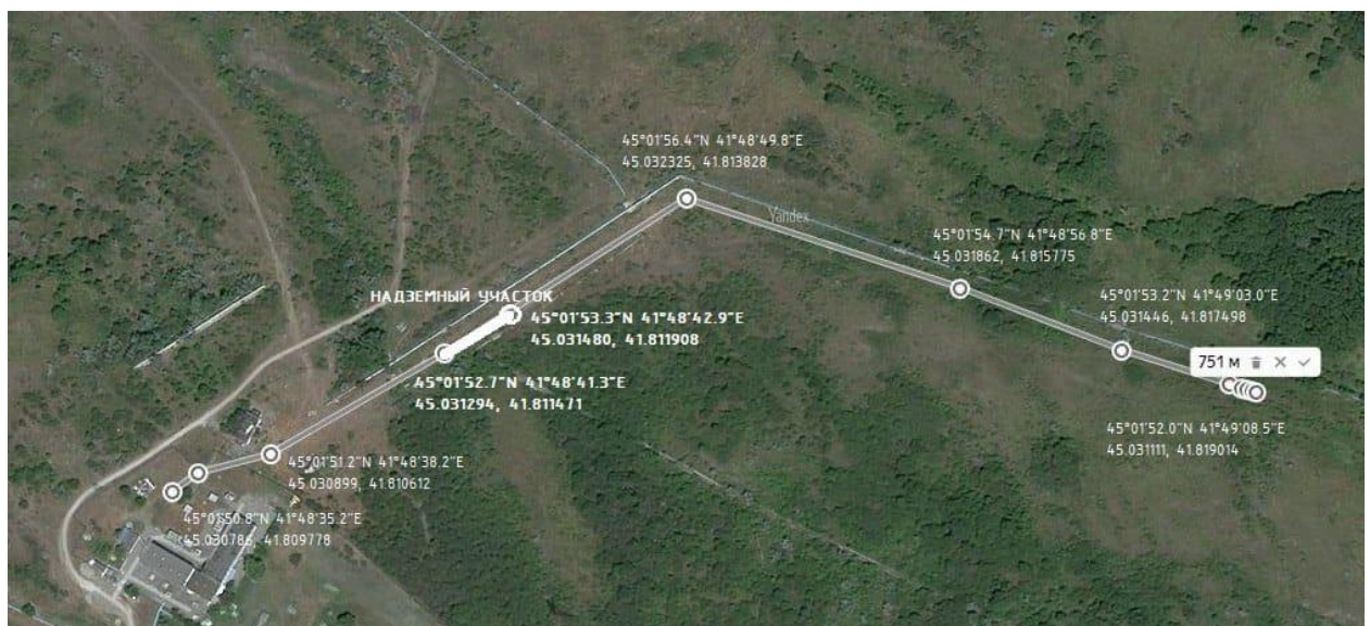
Рисунок 1.2. Ситуационный план с участком капитального ремонта водовода
